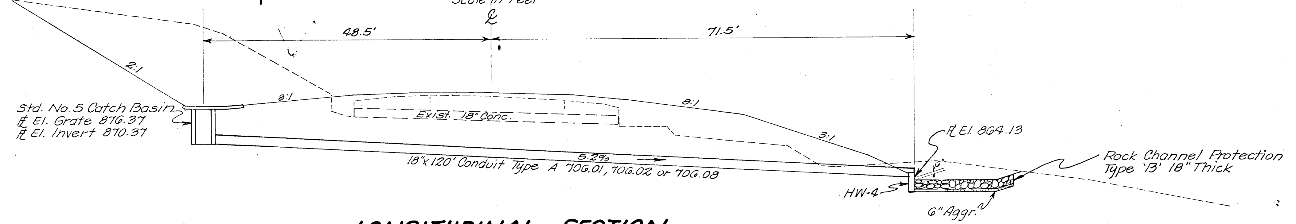
LONGITUDINAL SECTION
