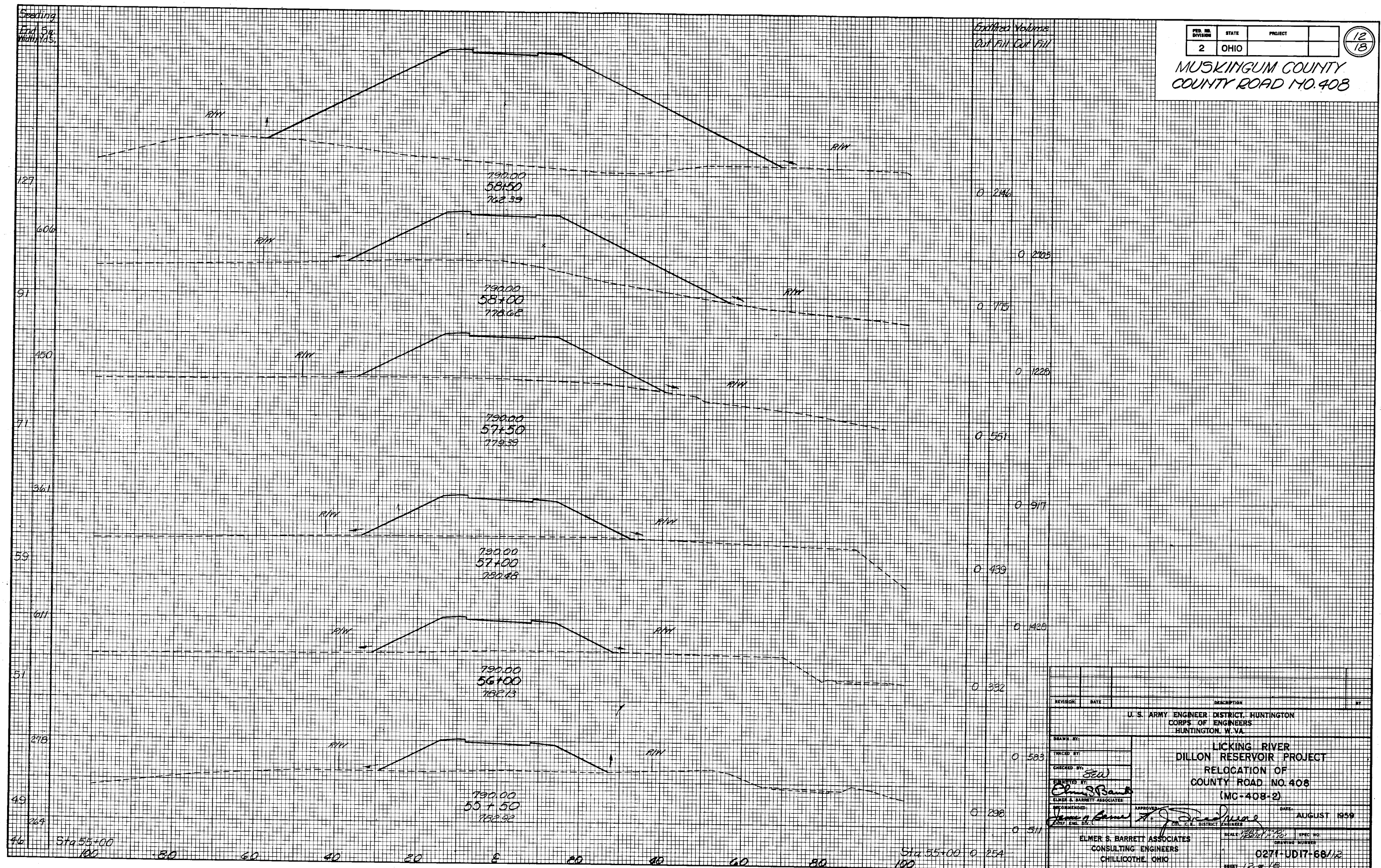
CROSS SECTIONS - STA. 55+50 TO STA. 58+50
