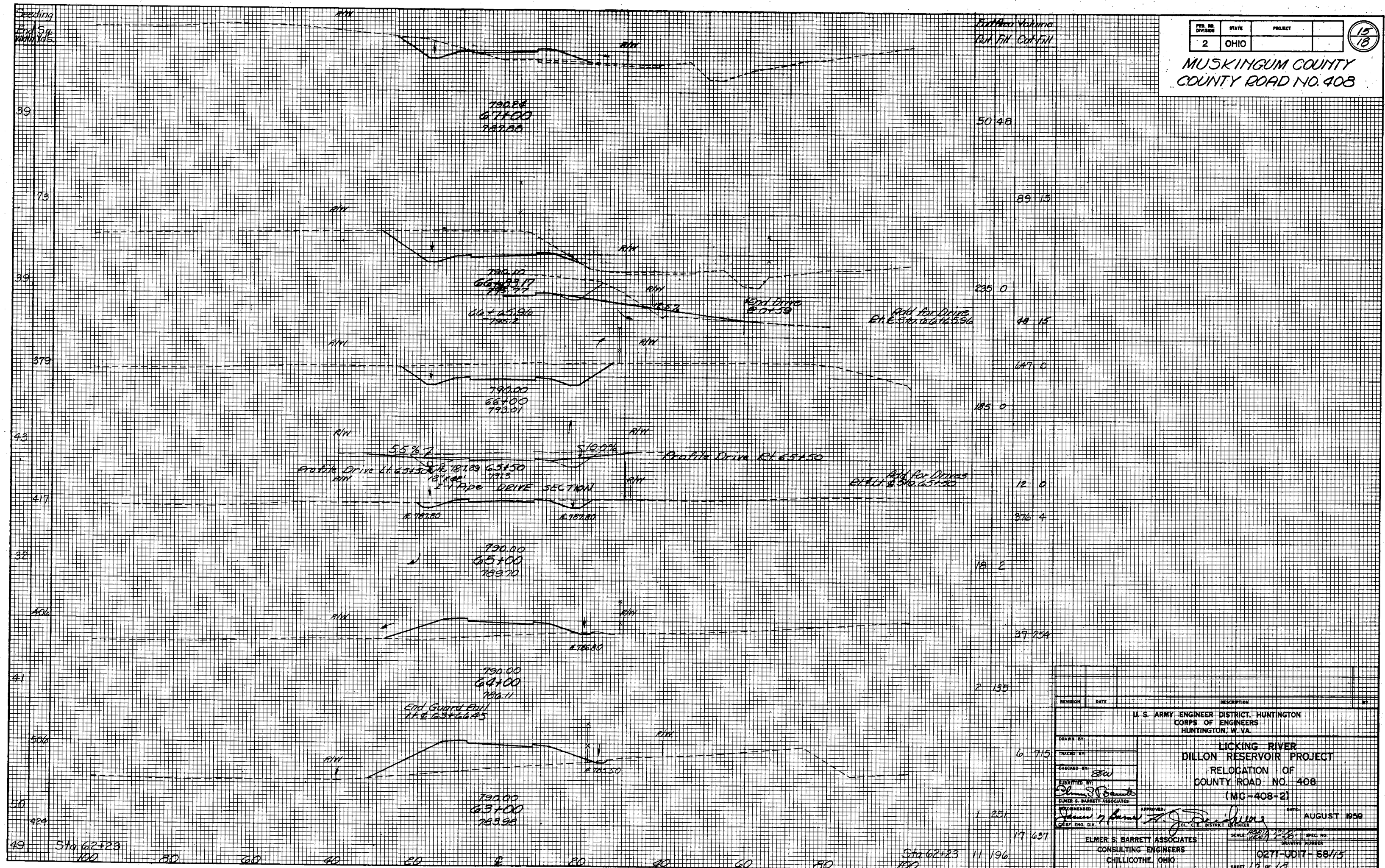
CROSS SECTIONS - STA. 63+00 TO STA. 67+00
