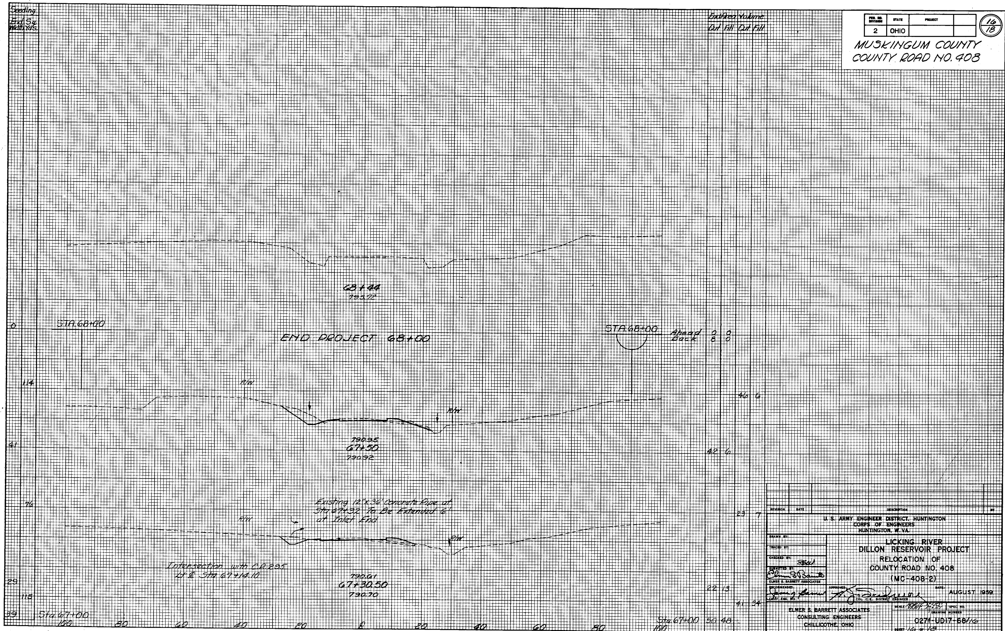
CROSS SECTION 15 - STA. 67+30.50 TO STA. 68+44
