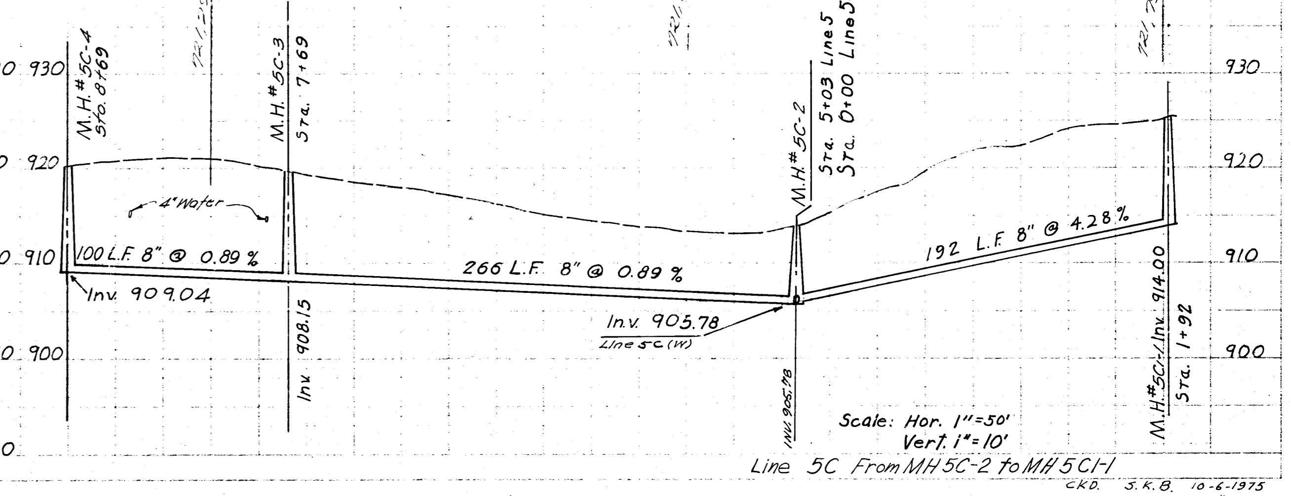
SEWER LINE 5-C M.H.#5C-2-M.H.#5C-1
